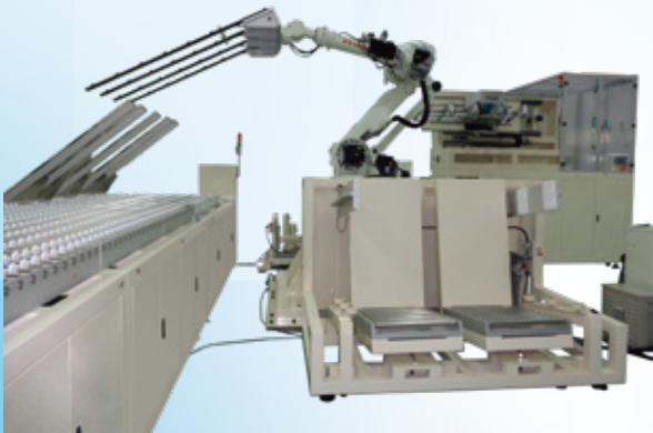
L-RACK 放板機 (DENSE UNPACK)
